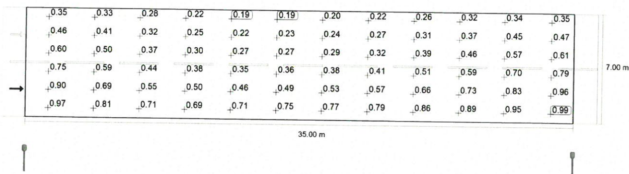
Observator 1: Valoarea de întreținere, densitatea luminii cu carosabil uscat [ \text{cd}/\text{m}^2 ] (Raster valoric)
